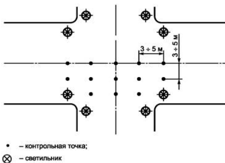
Рисунок А.6 - Расположение контрольных точек при измерении средней освещенности улиц на перекрестке
