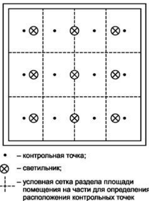
Рисунок А.3 - Расположение контрольных точек при измерении средней освещенности в помещении
