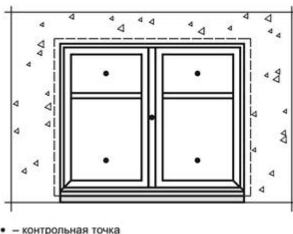
Рисунок А.8 - Расположение контрольных точек на внешней поверхности окна при измерении вертикальной освещенности (уровня засветки окон)
