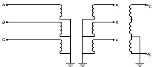
Рисунок Б.4 - Схема включения однофазных заземляемых трехобмоточных трансформаторов в трехфазных сетях с изолированной нейтралью и напряжением 3-35 кВ
