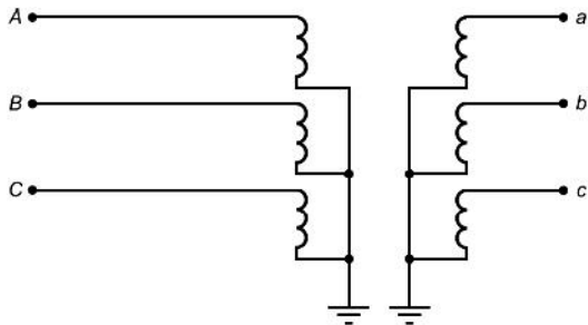
Рисунок Б.2 - Схема включения однофазных заземляемых и трехфазных заземляемых двухобмоточных трансформаторов в трехфазных сетях с изолированной нейтралью и напряжением 3-35 кВ
