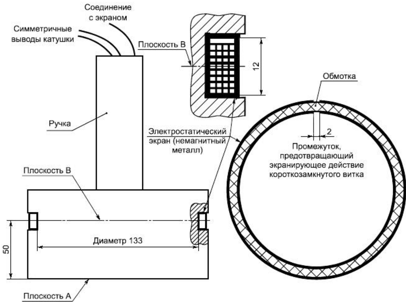
Рисунок А.1 - Конструкция рамочного датчика
