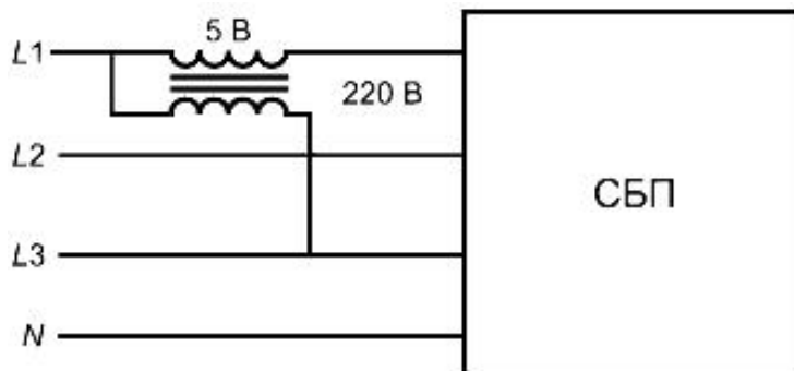
Рисунок D.2 - Фазовая несимметрия
