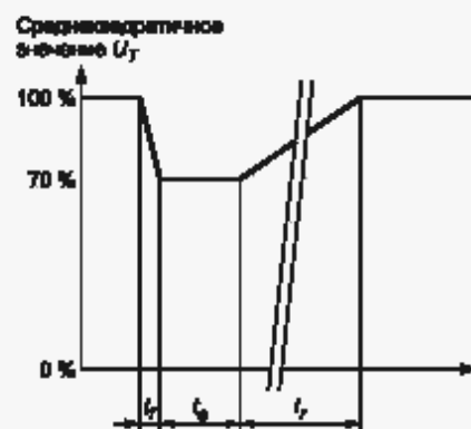
Рисунок 3 — Изменение напряжения
