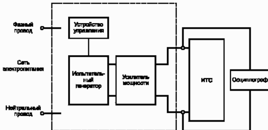
б) Схема испытаний с использованием усилителя мощности
