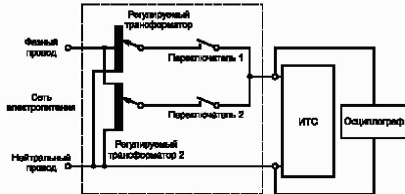
а) Схема испытаний с использованием регулируемых трансформаторов и переключателей
