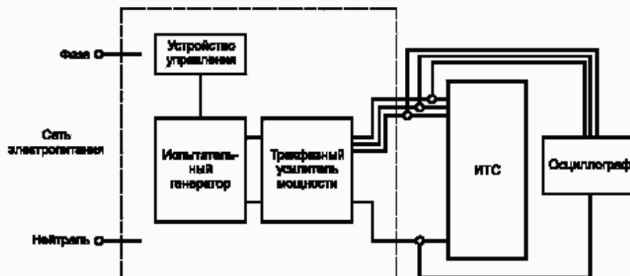
Рисунок С.2 — Схема установки для испытаний трехфазных систем при воздействии провалов, кратковременных прерываний и изменений напряжения электропитания
